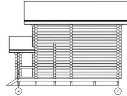
Фасад A-E
