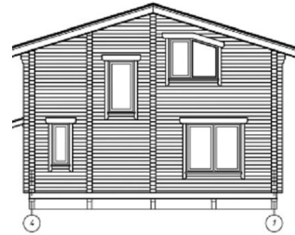
Фасад 4-1
