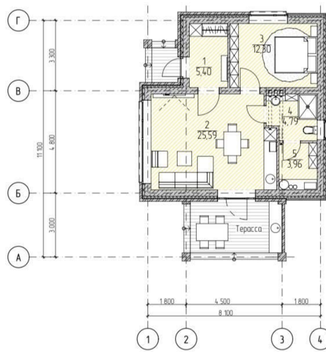
План 1-го этажа с расстановкой мебели и оборудования М175
